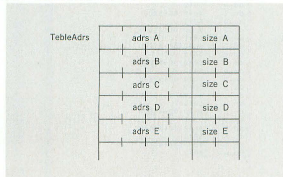
図3 _DMA_MOV_Aが使用するチェーンテーブル
